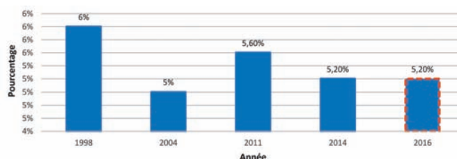
Figure 36 : Evolution du pourcentage des enfants de moins de cinq ans présentant une émaciation de 1998 à 2016
